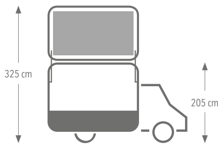
Ausschankklappe: b 194 cm x h 117,5 cm
